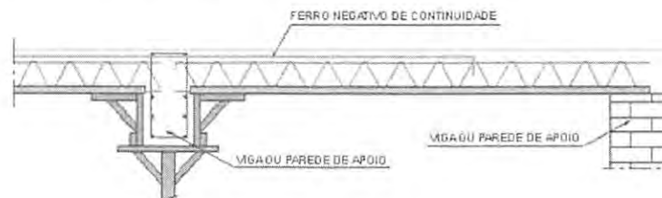
Imagem 2-Posição da ferragem negativa
